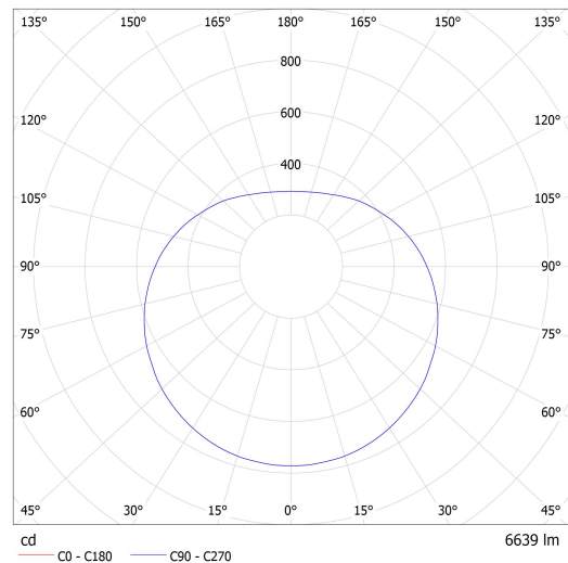
Luminaire: Lucis ZT.P3.500.X PE POLARIS ZT PE LED Lamps: 1 x LED G6
