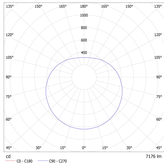
Lucis ZT.P4.500.X PE POLARIS ZL PE LED / LDC (Polar)
