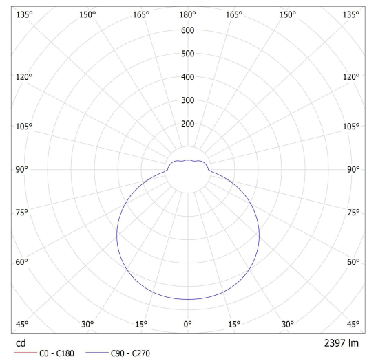
Lucis S33.K4.TEZ3 TENDO LED / LDC (Polar)
