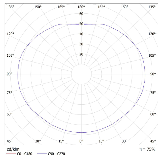
Luminaire: Lucis ZK2.11.GB.61R GEO Lamps: 1 x HALOPIN ECO 48W
