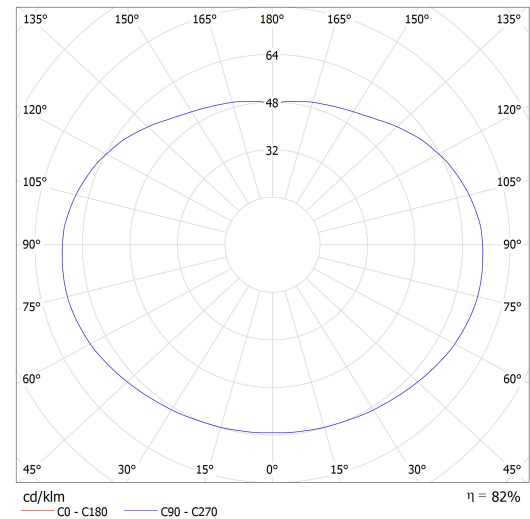
Lucis ZK.11.200.X POLARIS ZK / LDC (Polar)
