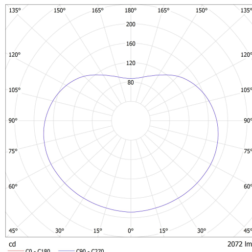
Lucis ZKS.P2.200.X POLARIS ZKS.P LED / LDC (Polar)
