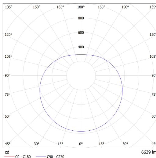
Lucis ZT.P1.600.X PE POLARIS ZT PE LED / LDC (Polar)
