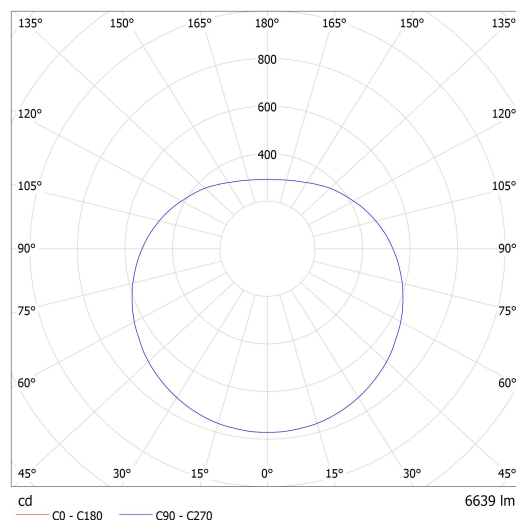
Lucis ZL1.P1.600.X PE POLARIS ZL PE LED / LDC (Polar)
