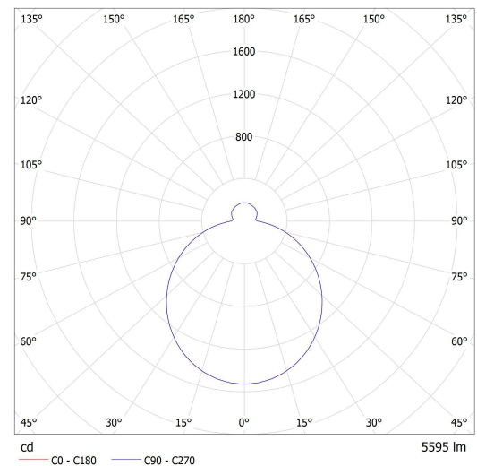
Lucis ZL3.K2.O50 PE FORUM PE LED / LDC (Polar)
