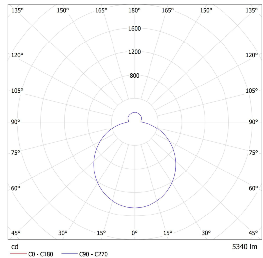
Lucis PS43.K1.O50 PE FORUM PE LED / LDC (Polar)
