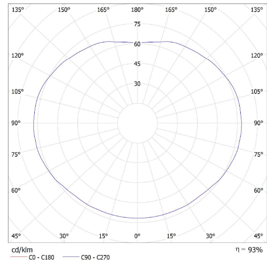
Luminaire: Lucis ZT.11.300.X POLARIS ZT Lamps: 1 x Osram 100W
