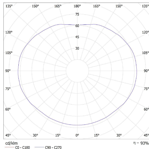
Lucis ZK.11.400.X POLARIS ZK / LDC (Polar)
