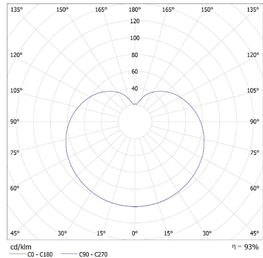
Lucis ZK.11.500.X PE POLARIS ZK PE / LDC (Polar)
