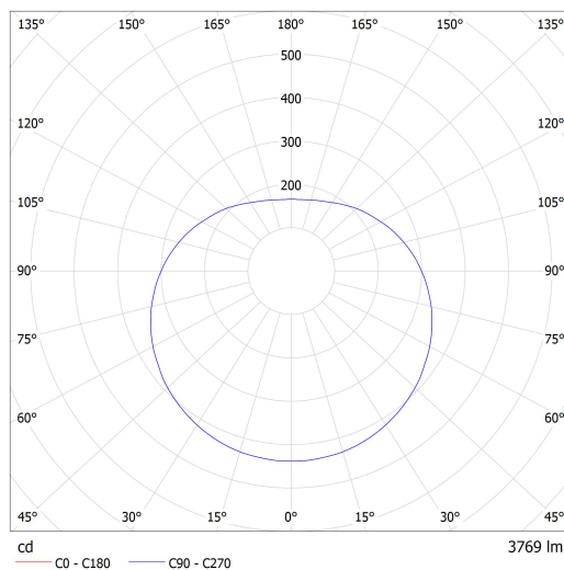
Lucis ZL1.P2.400.X PE POLARIS ZL PE LED / LDC (Polar)
