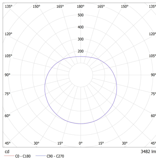
Lucis ZT.P1.400.X PE POLARIS ZT PE LED / LDC (Polar)
