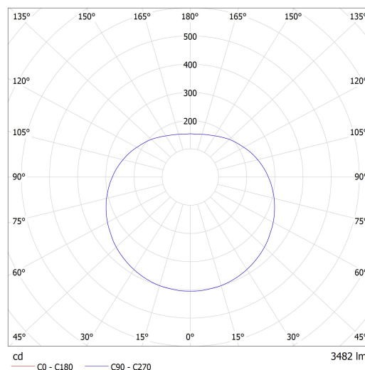
Luminaire: Lucis ZT.P1.400.X PE POLARIS ZT PE LED Lamps: 1 x LED G6
