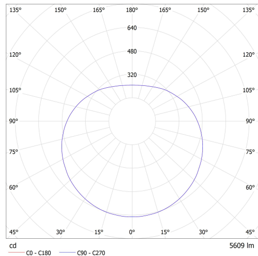
Lucis ZT.P2.500.X PE POLARIS ZT PE LED / LDC (Polar)
